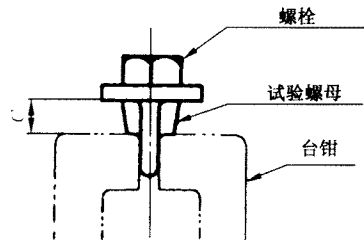
图 4 固定螺母法
