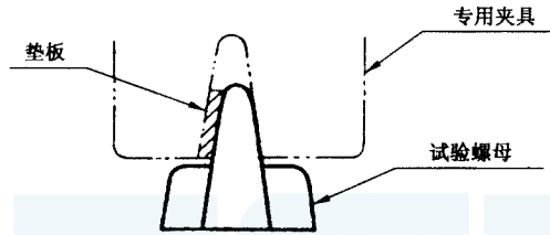
图 2 专用夹具
