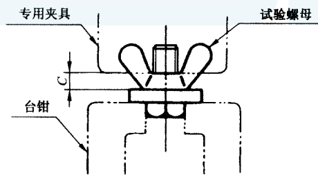
图 3 固定螺栓法
