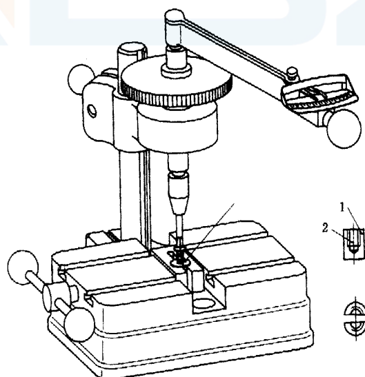
1—开合模；2—盲孔
