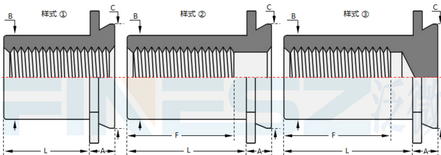
CSS样式:
